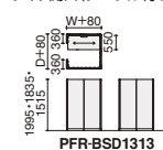
サイド開口(テーブル付き)
